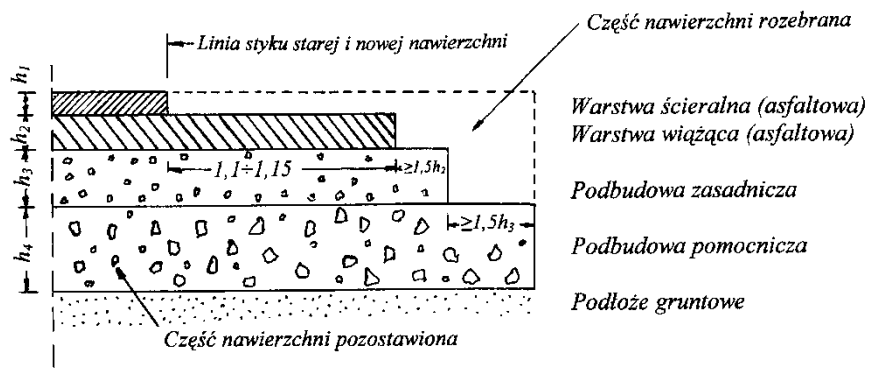
Rys. 2. Konstrukcja połączenia starej i nowej nawierzchni
